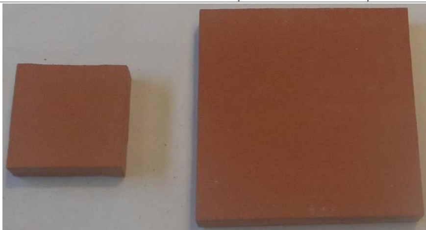
Figura 2. Riproduzione fotografica di provini di dimensioni 5 x 5 cm e 10 x 10 cm ricavati per taglio da una tegola tal quale del prodotto “Tegola Rosso Naturale”. Su tali provini sono state effettuate le determinazioni sperimentali oggetto del presente rapporto.
