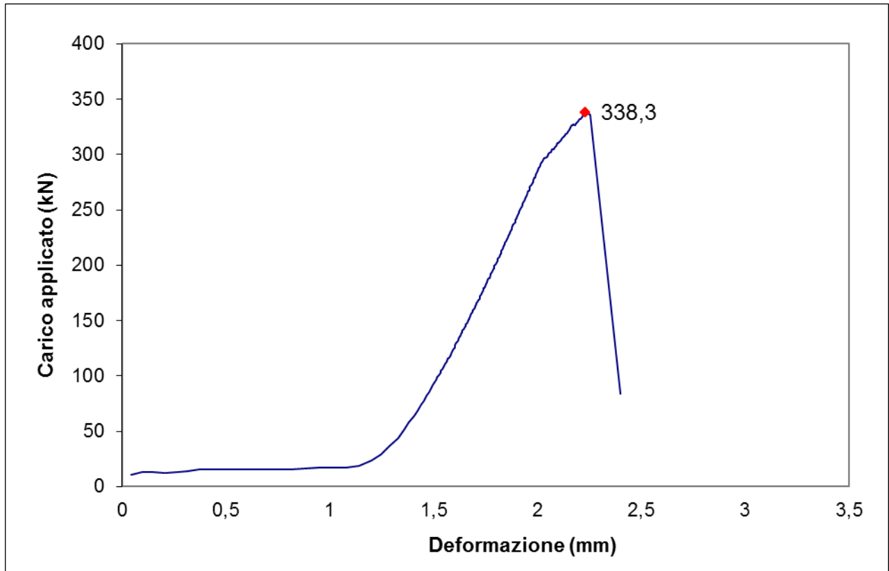
Figura 2. “Forato 8x24x33”: diagramma di compressione del provino n. 2 (orientamento dell’elemento rispetto al carico: fori orizzontali. Dimensioni nominali della faccia testata: 330 x 80 mm).
